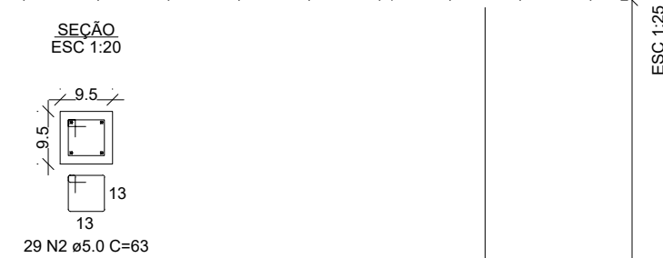
P32 PAVIMENTO - COBERTURA - L2
