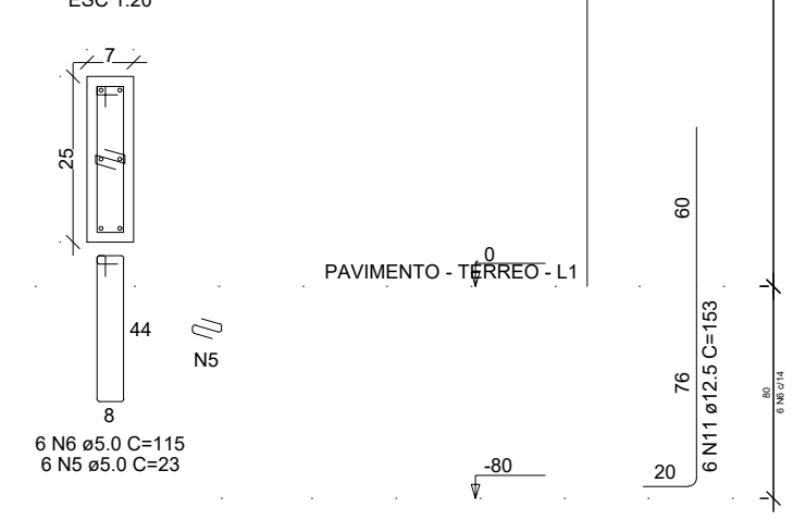
PAVIMENTO - TÉRREO - L1
