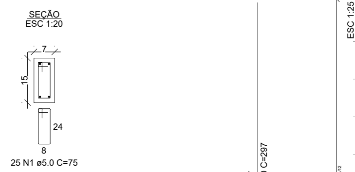
P25 PAVIMENTO - COBERTURA - L2
