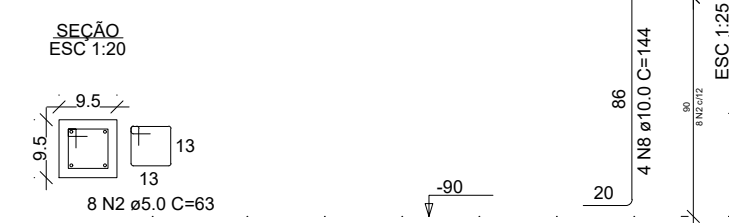
PAVIMENTO - TÉRREO - L1
