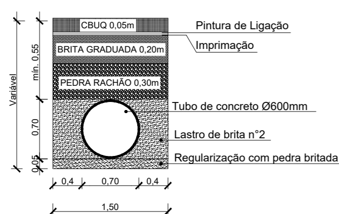
DETALHE 06 SEÇÕES DE ESCAVAÇÃO E REATERRO P/TUBULAÇÃO SEM ESCALA
