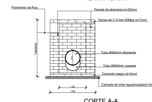
DETALHE 05 CAIXA COLETORA 120cmx120cm SEM ESCALA
