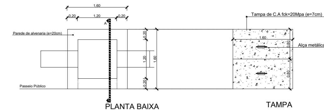
PLANTA BAIXA
