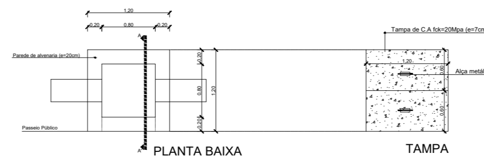
PLANTA BAIXA
