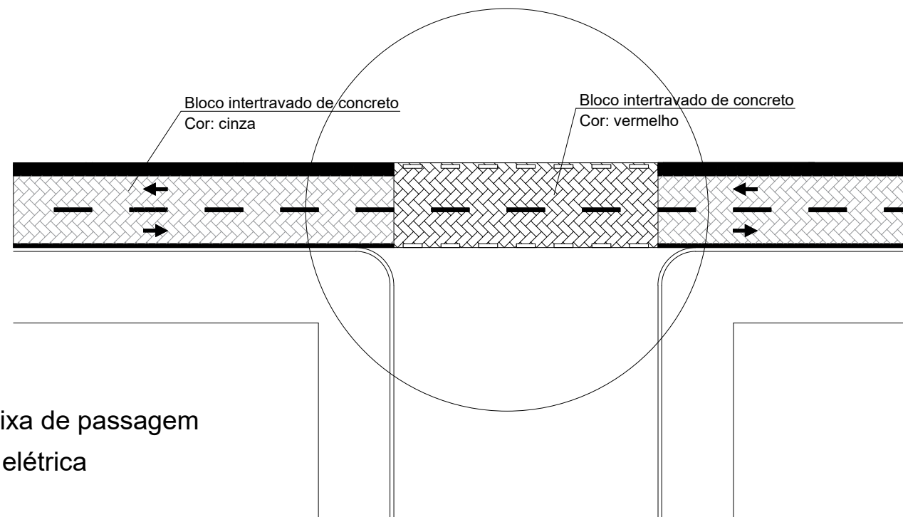
PLANTA BAIXA - Cruzamento com rua S/ESCALA
