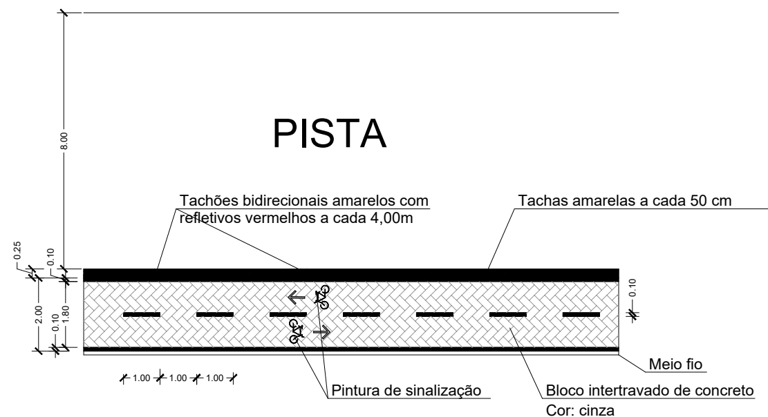
PLANTA BAIXA S/ESCALA
