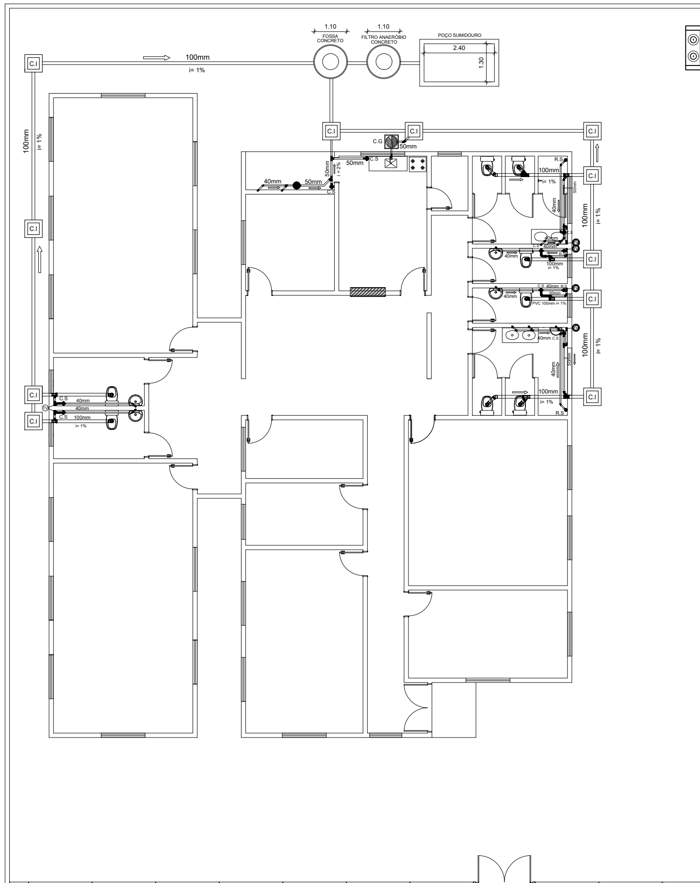
PLANTA BAIXA SANITÁRIA
