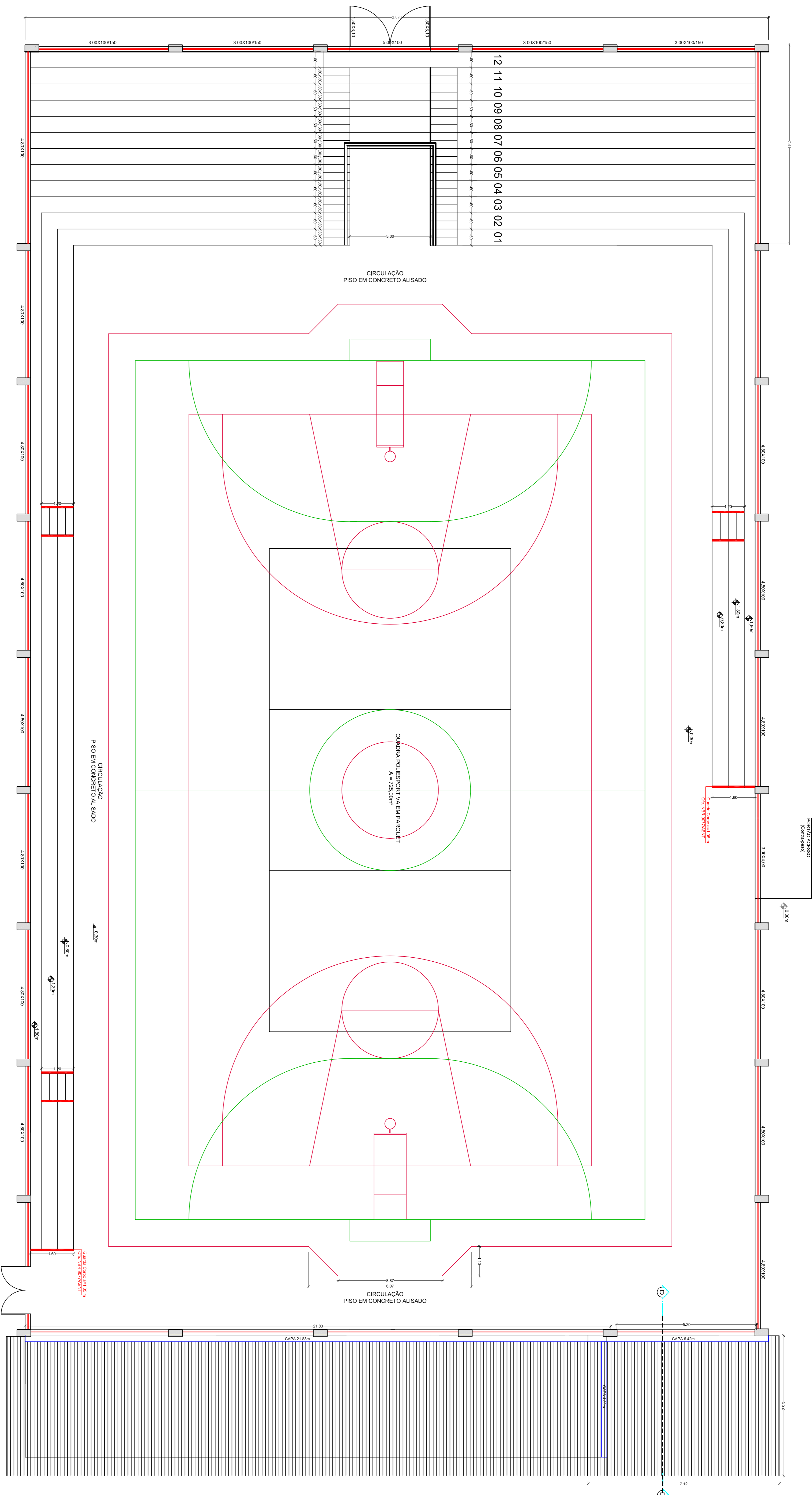
PLANTA BAIXA
